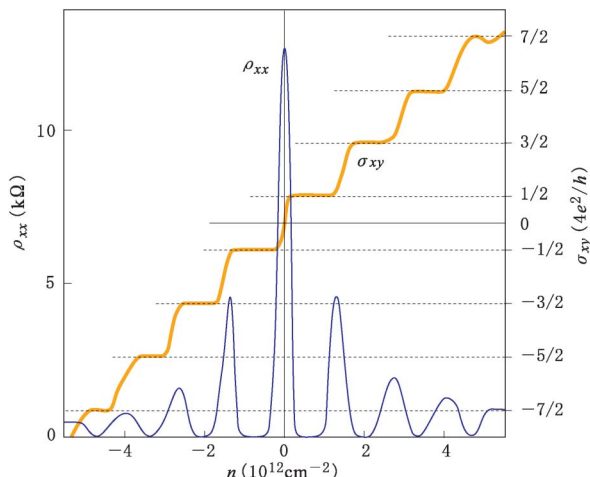
第10図 観測されたグラフェンのホール伝導度 1)
